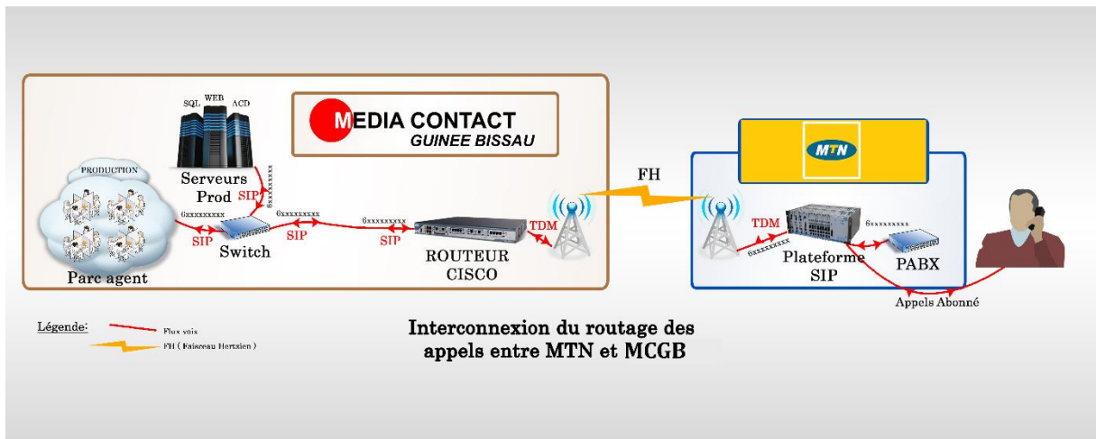
Figure 1 : Architecture de routage des appels
