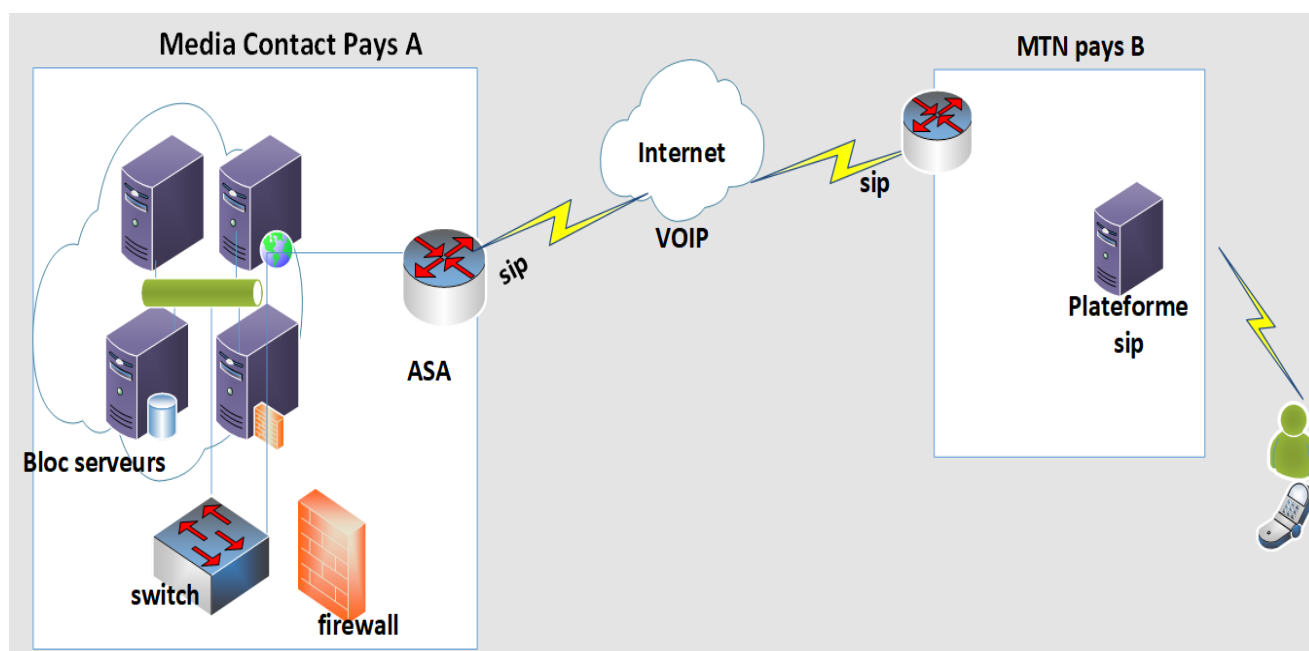
Architecture d'interconnexion trunk SIP avec MTN pays B
